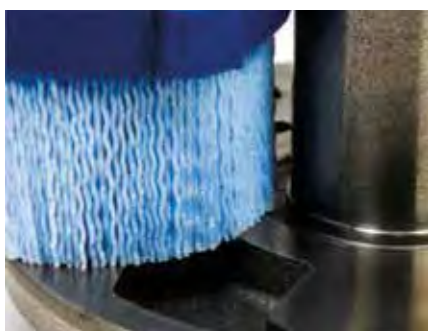
Spazzola a disco per la finitura di stampati in ghisa / Disc brush for cast iron finishing
