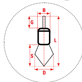
P10 punta Acciaio ottonato / Brass Plated Steel
